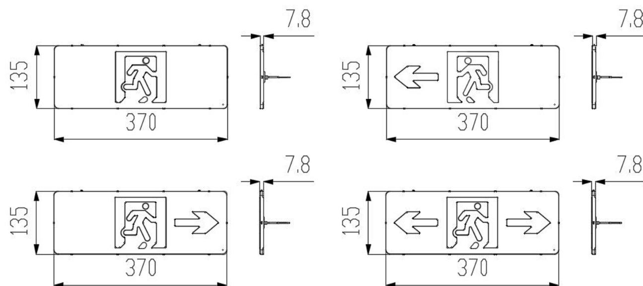
图 1-1 A23-B 双面产品外形图
