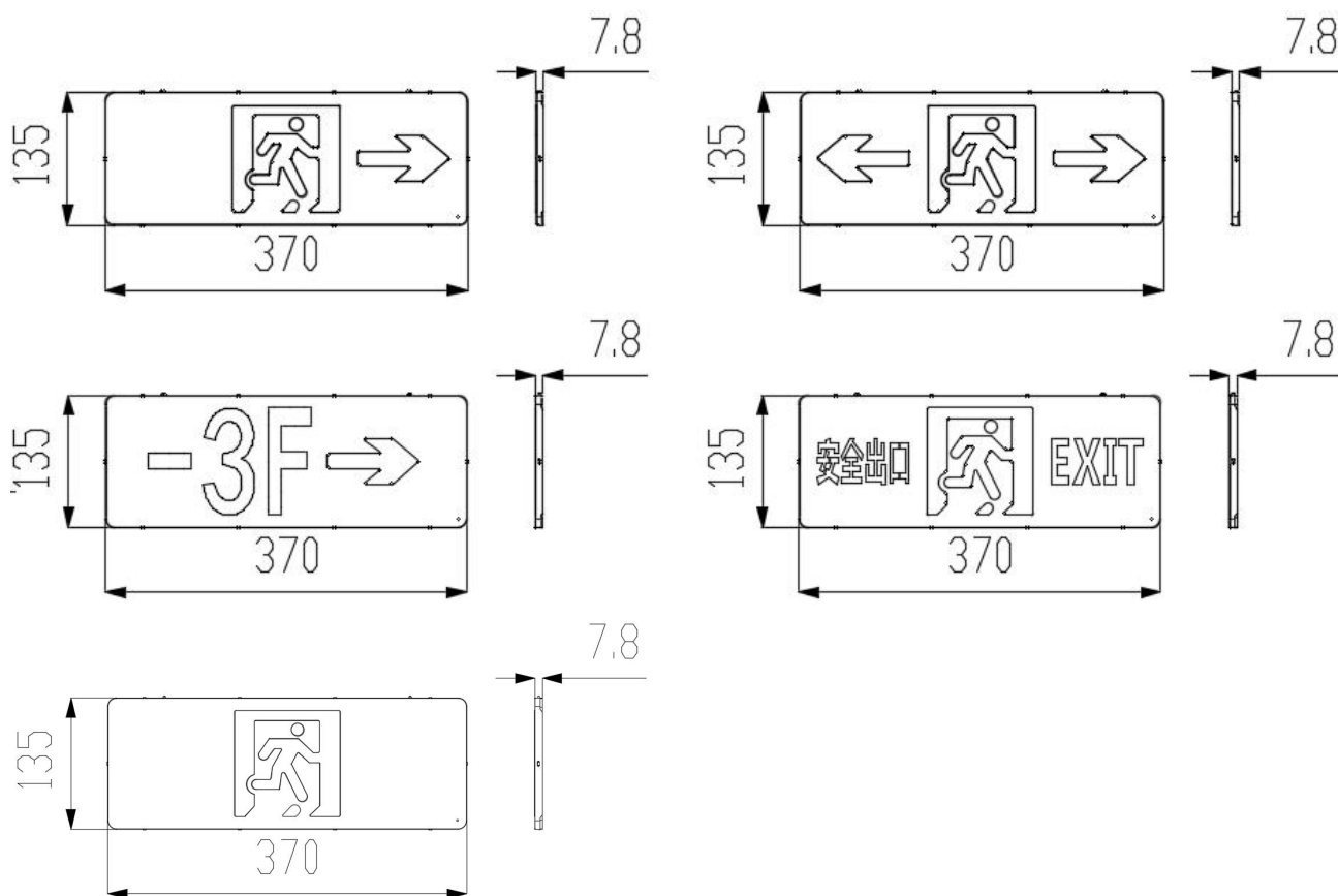
图 1-1 A23-B 双面产品外形图
