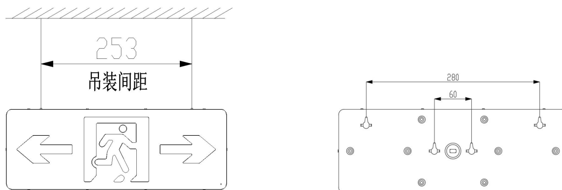
图 4 安装示意图
