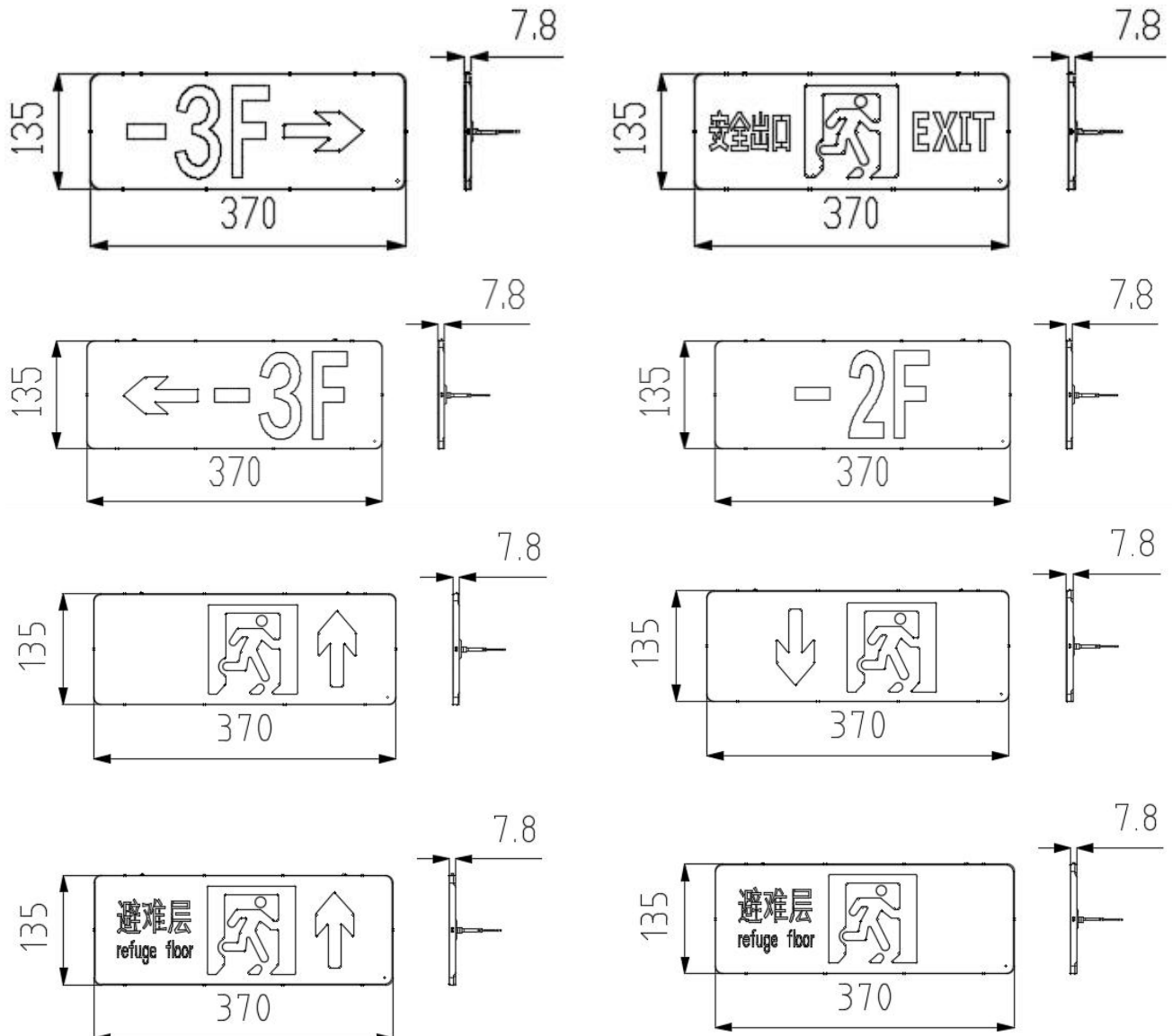
图 1-2 A23-B 单面产品外形图
