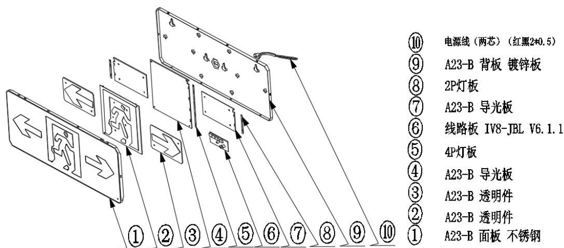
图 2-2 A23-B 单面结构图
