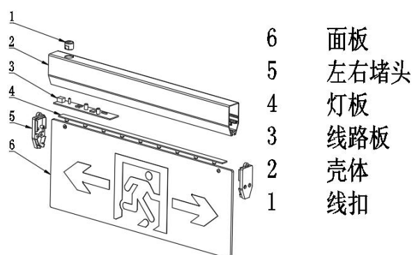
图 2 ZA05 系列结构图
