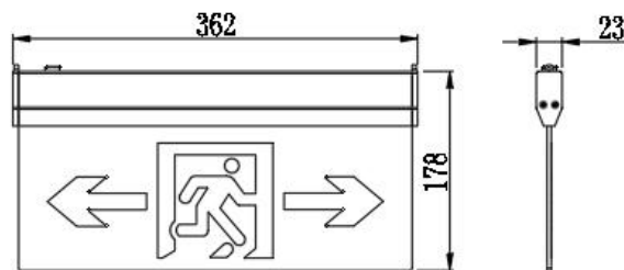
图 1 ZA05 系列产品外形图
