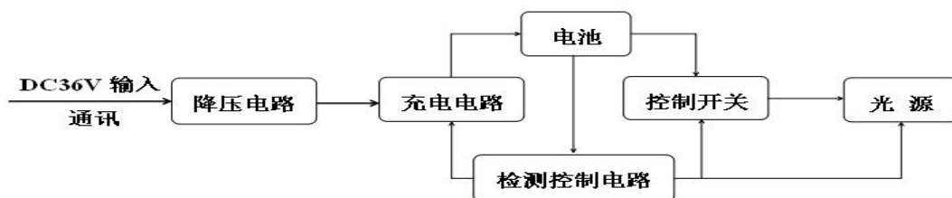
图 3 系统工作原理图
