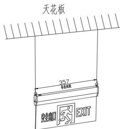
图 4 安装示意图
